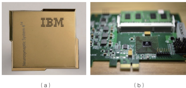
图1 IBM 研制的“TrueNorth”芯片(a)和中科院计算所研制的“寒武纪”芯片及其板卡(b)
